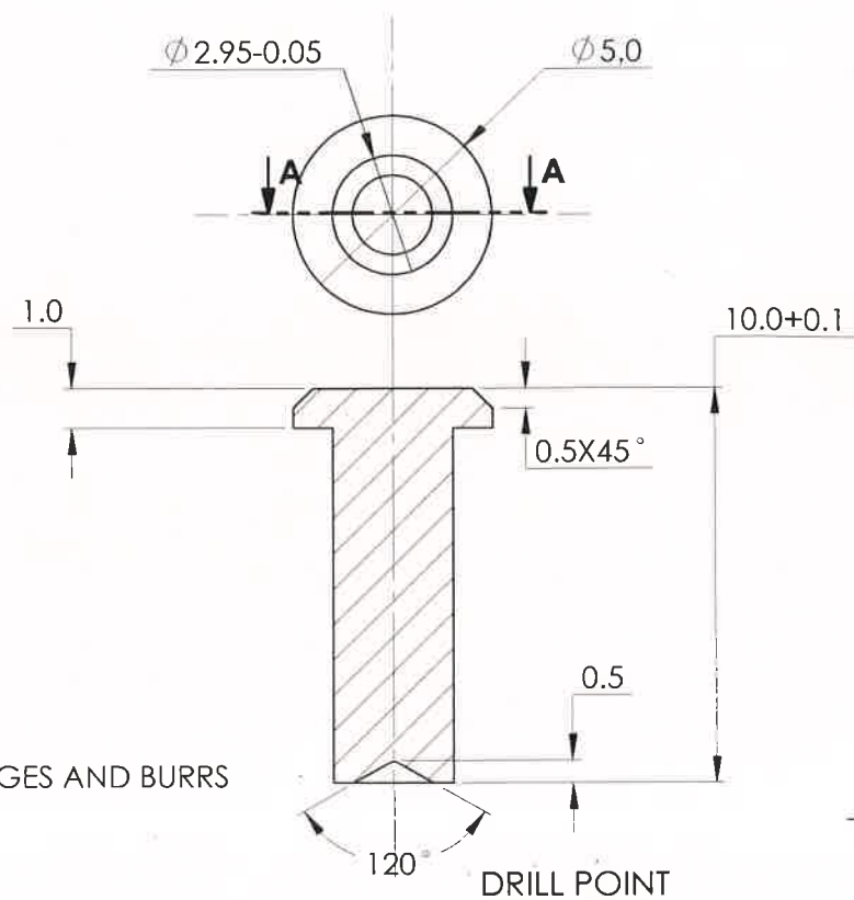
SECTION A-A
