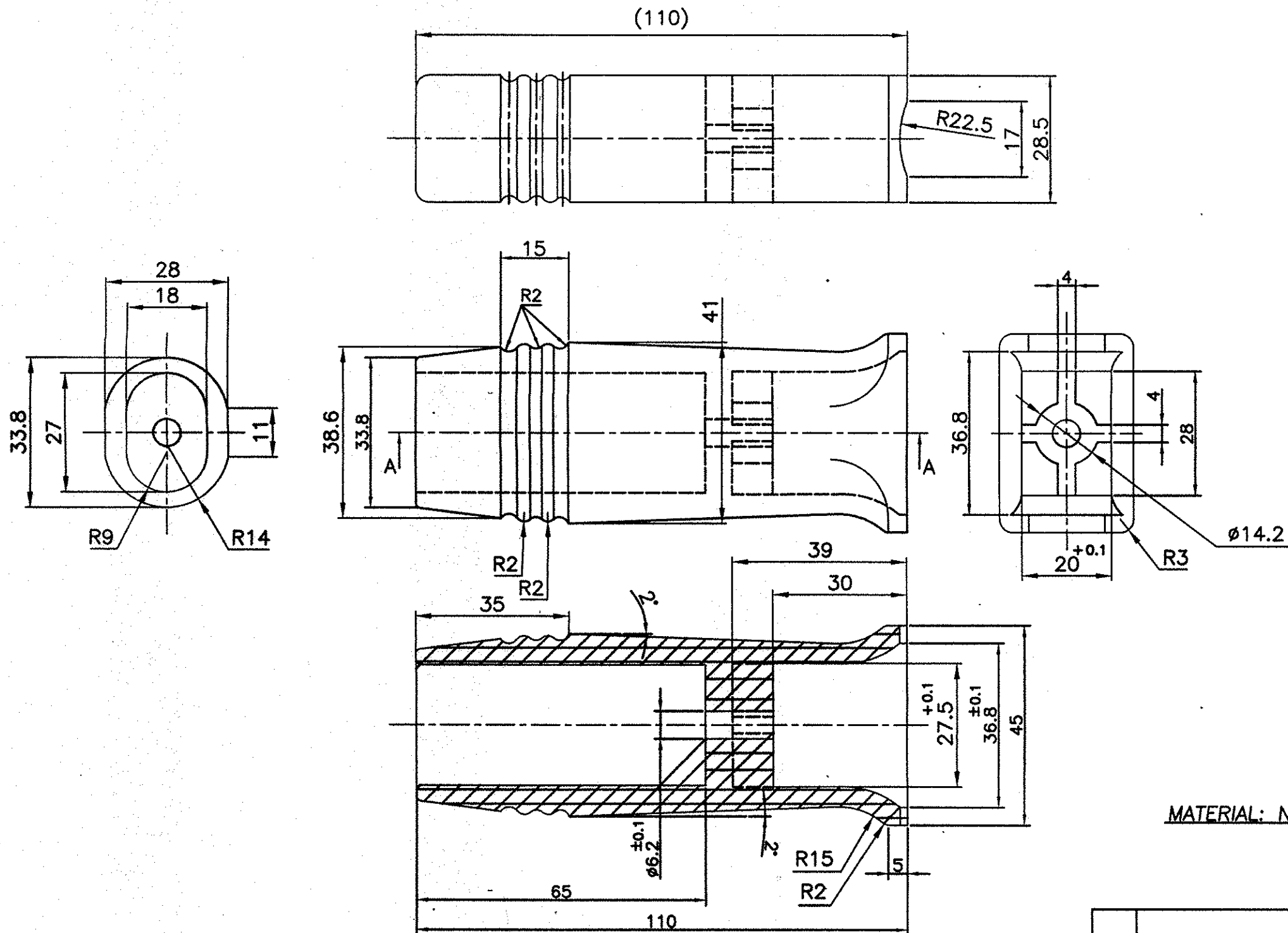
SECTION - A-A
