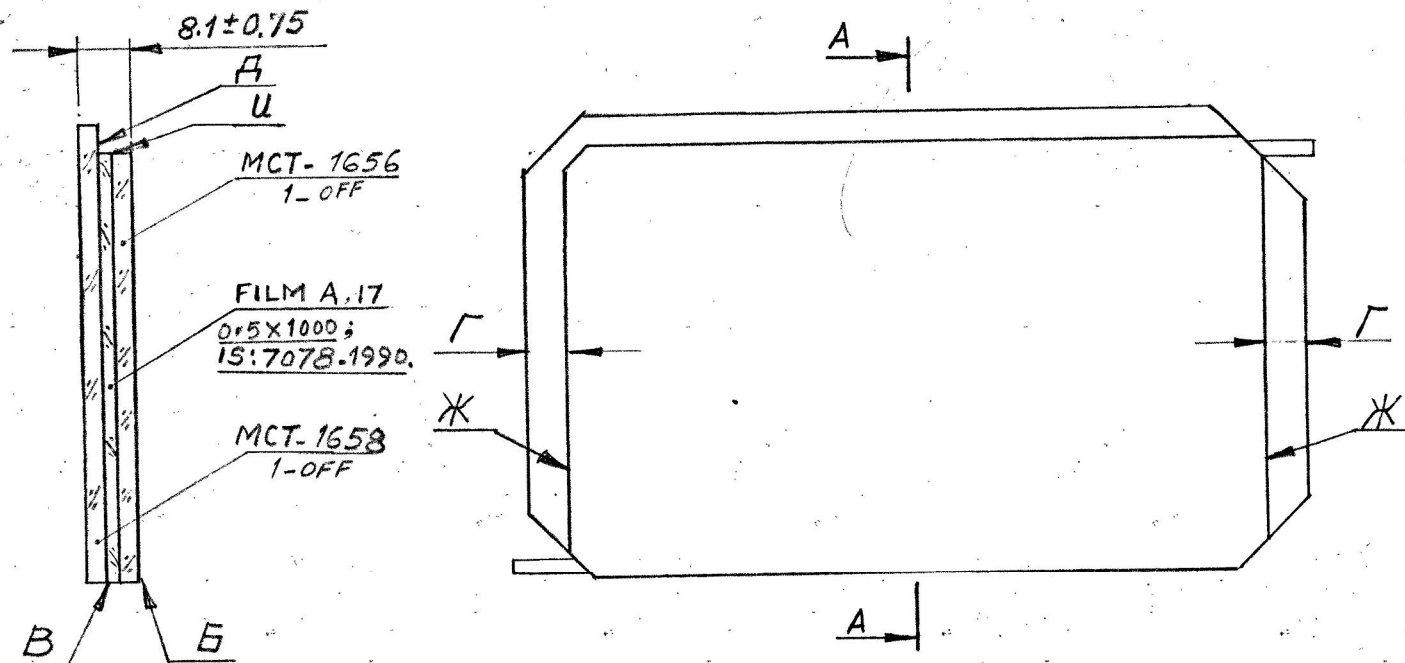
SEC. A-A.
