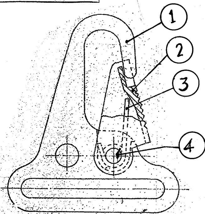
HOOK ASSY, PER GUN 2 NOS.
