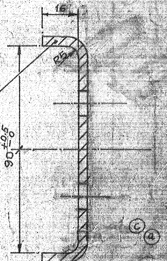
SECTION - A-A
