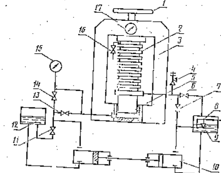
SCHEMATIC OF AUTOCLAVE TYPE AP-2 Схема аппарата типа АП-2
