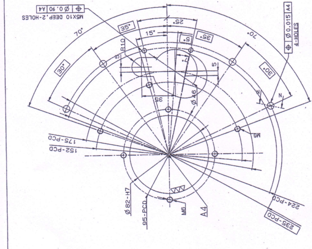
DETAIL-A4
