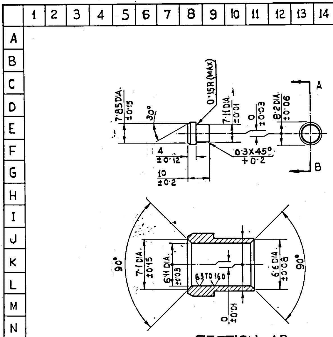
SECTION - AB SCALE: 3:1
