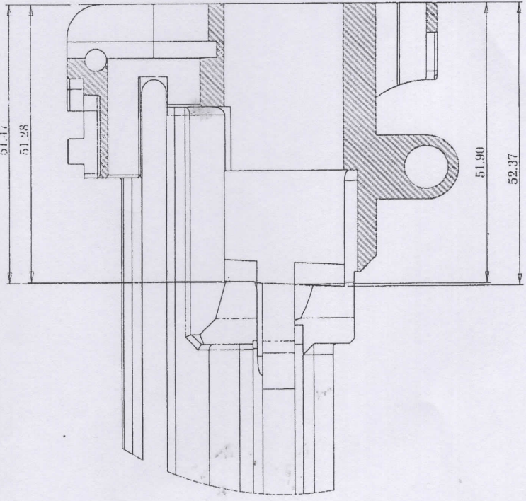
DETAIL Y SCALE 1:1
