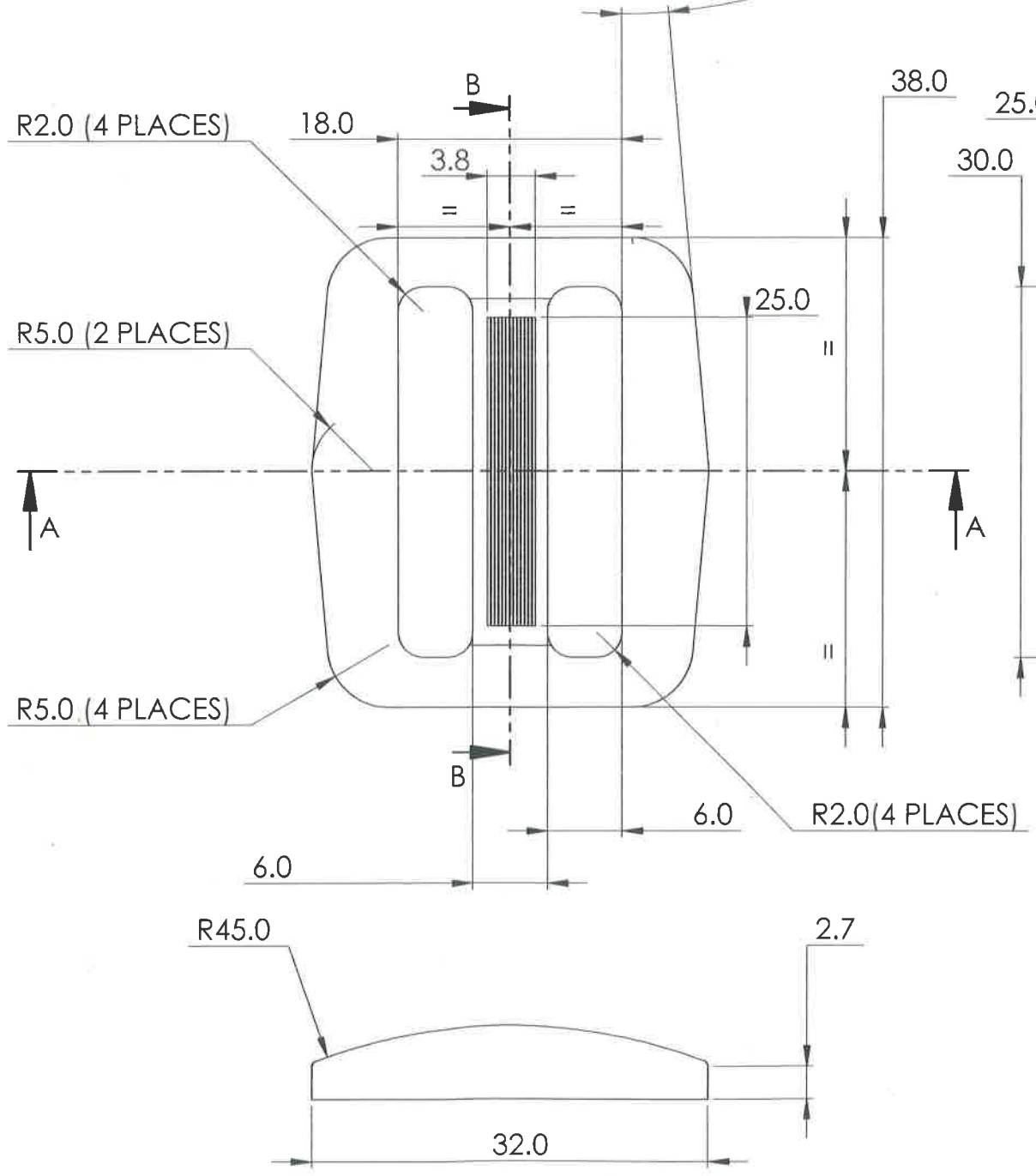
SECTION B-B SCALE 2:1
