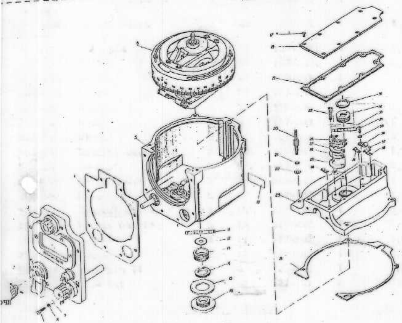
Fig. 2. ELECTRICAL DIRECTIONAL GYRO I27-C8. Рис. 2. Гироскоп компас электрический I27-06
