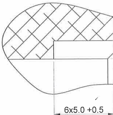
DETAIL-B SCALE-5:1
